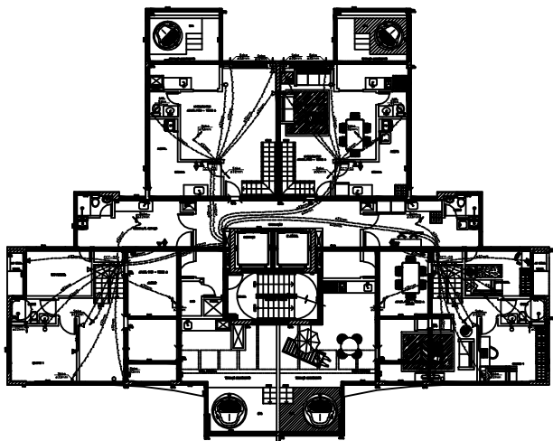
PLANTA BAIXA 17º PAV. TORRE-A INF. DUPLEX DEZ/75
