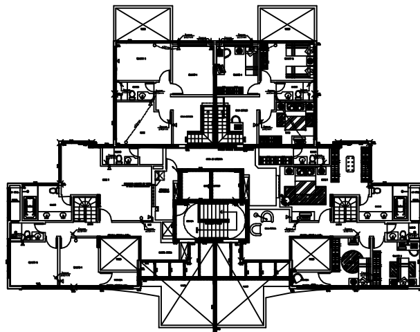
PLANTA BAIXA 18º PAV. TORRE-A SUP. DUPLEX DEZ/75
